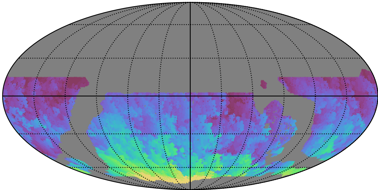
weather_cloudso2v3.4_10yrs WFD r band: Max HA
