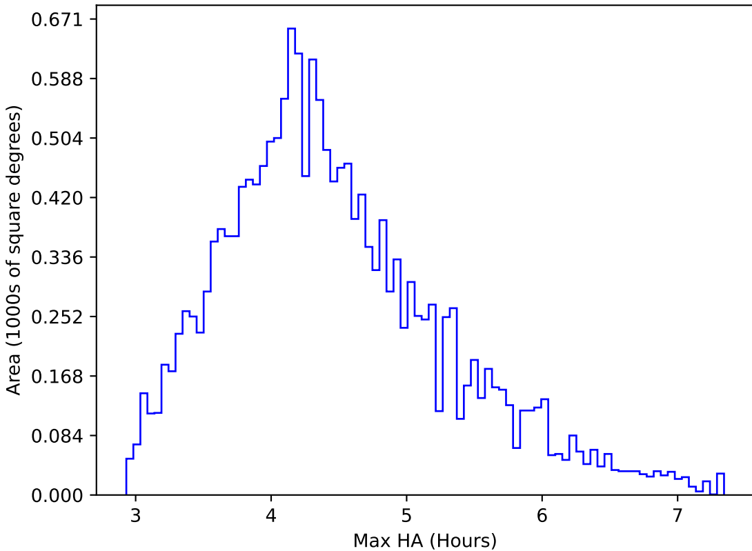
weather_cloudso2v3.4_10yrs WFD r band: Max HA
