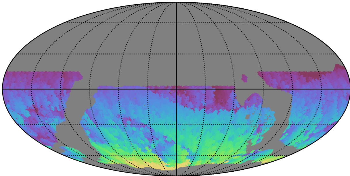
weather_cloudso2v3.4_10yrs WFD i band: Max HA
