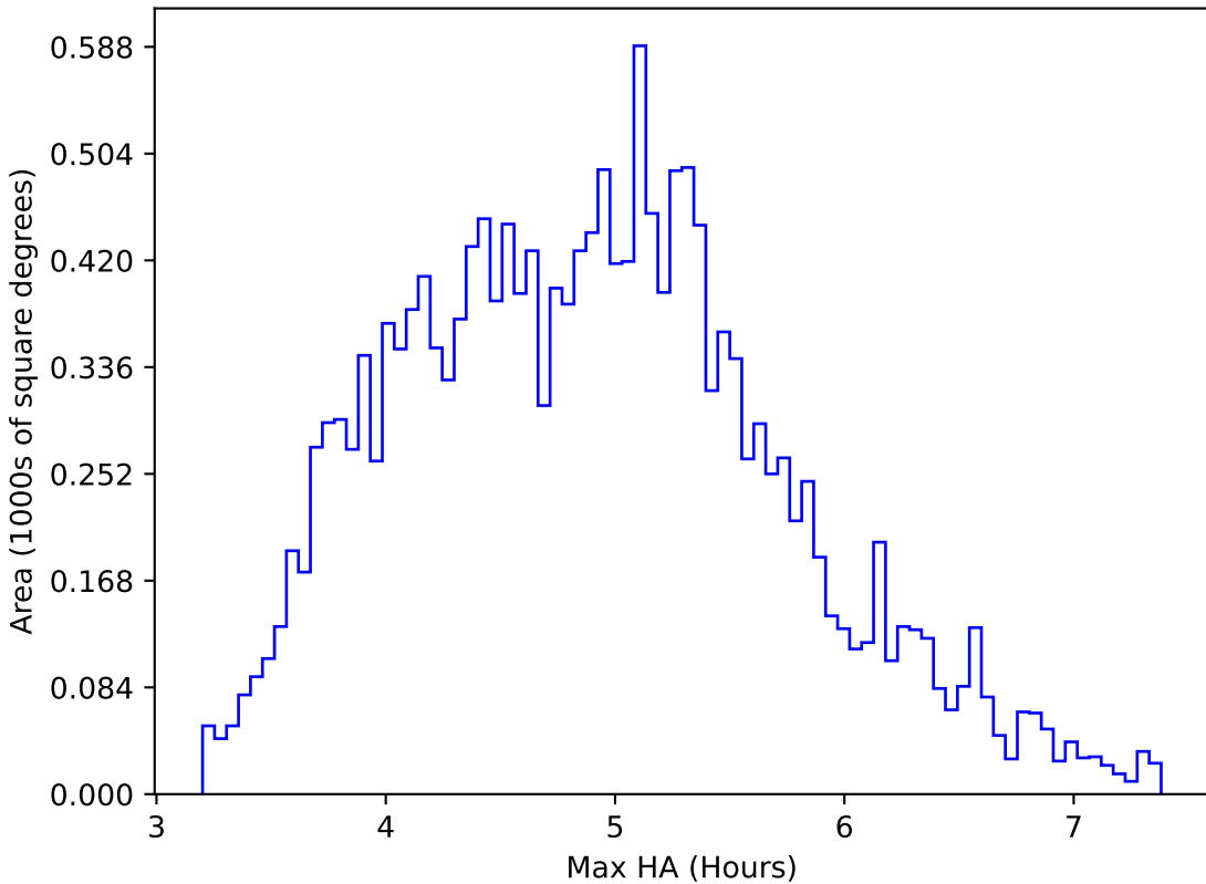
weather_cloudso2v3.4_10yrs WFD i band: Max HA
