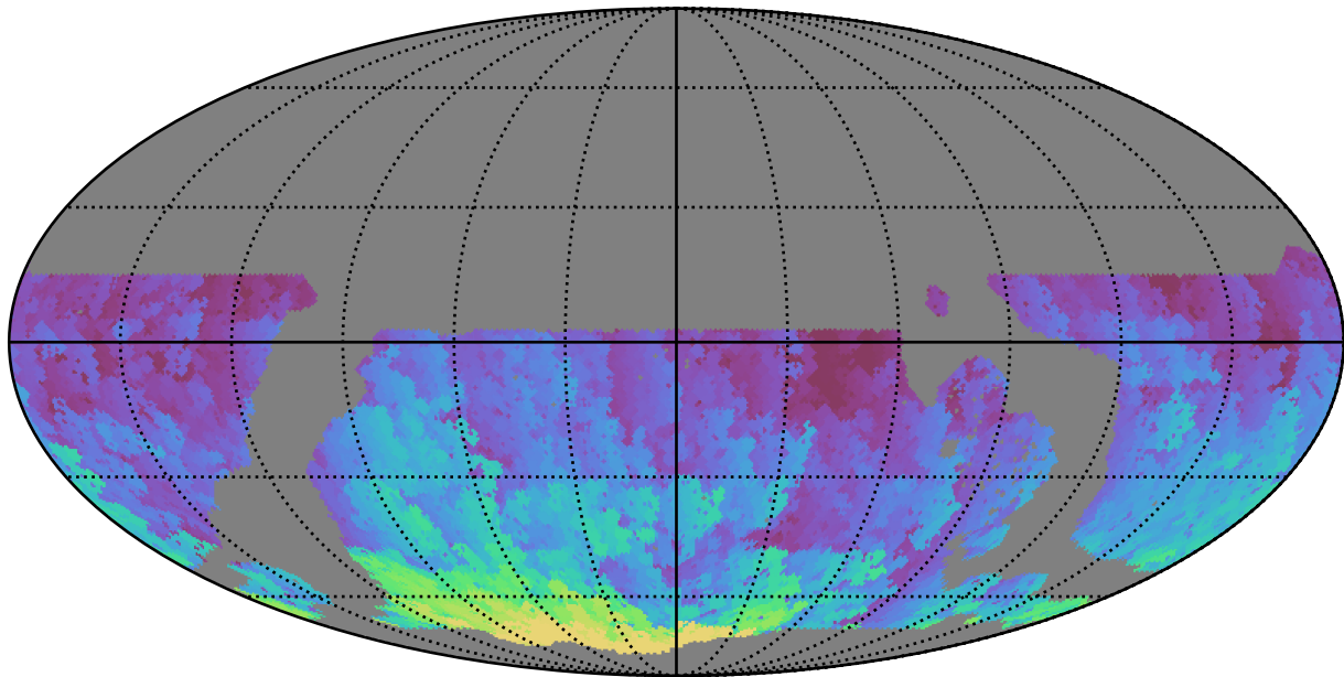
weather_cloudso2v3.4_10yrs WFD g band: Max HA
