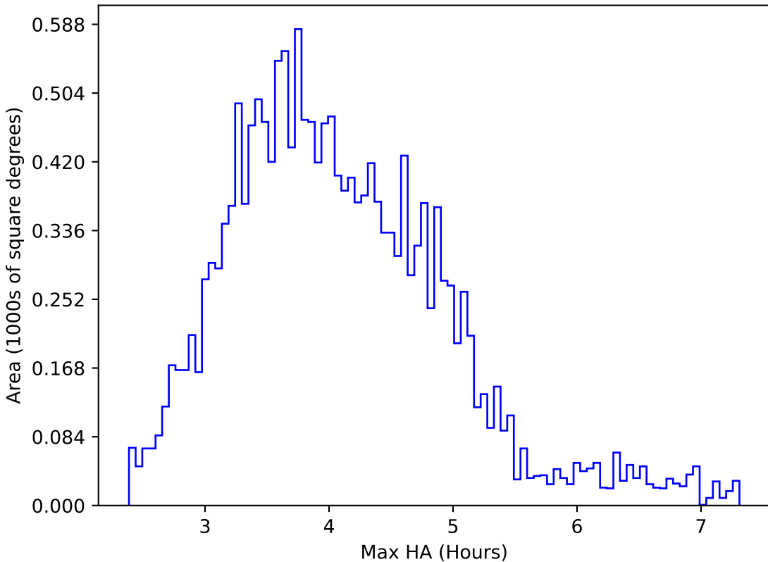
weather_cloudso2v3.4_10yrs WFD g band: Max HA
