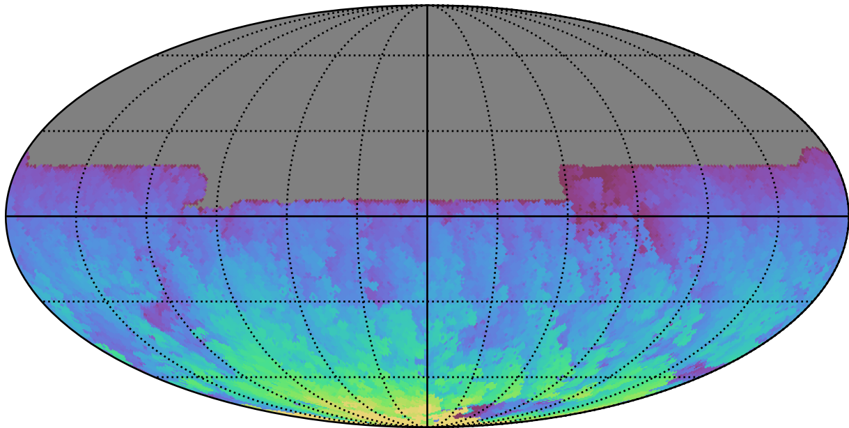
weather_cloudso2v3.4_10yrs All sky y band: Max HA
