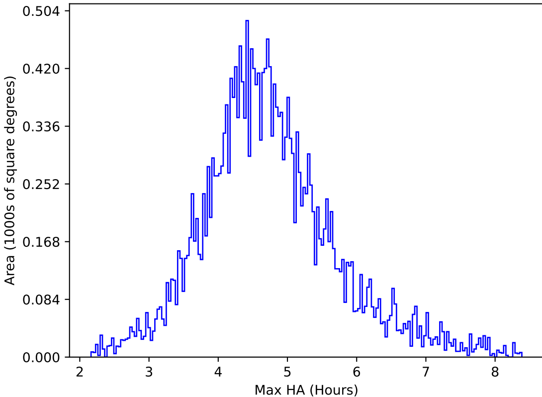
weather_cloudso2v3.4_10yrs All sky y band: Max HA
