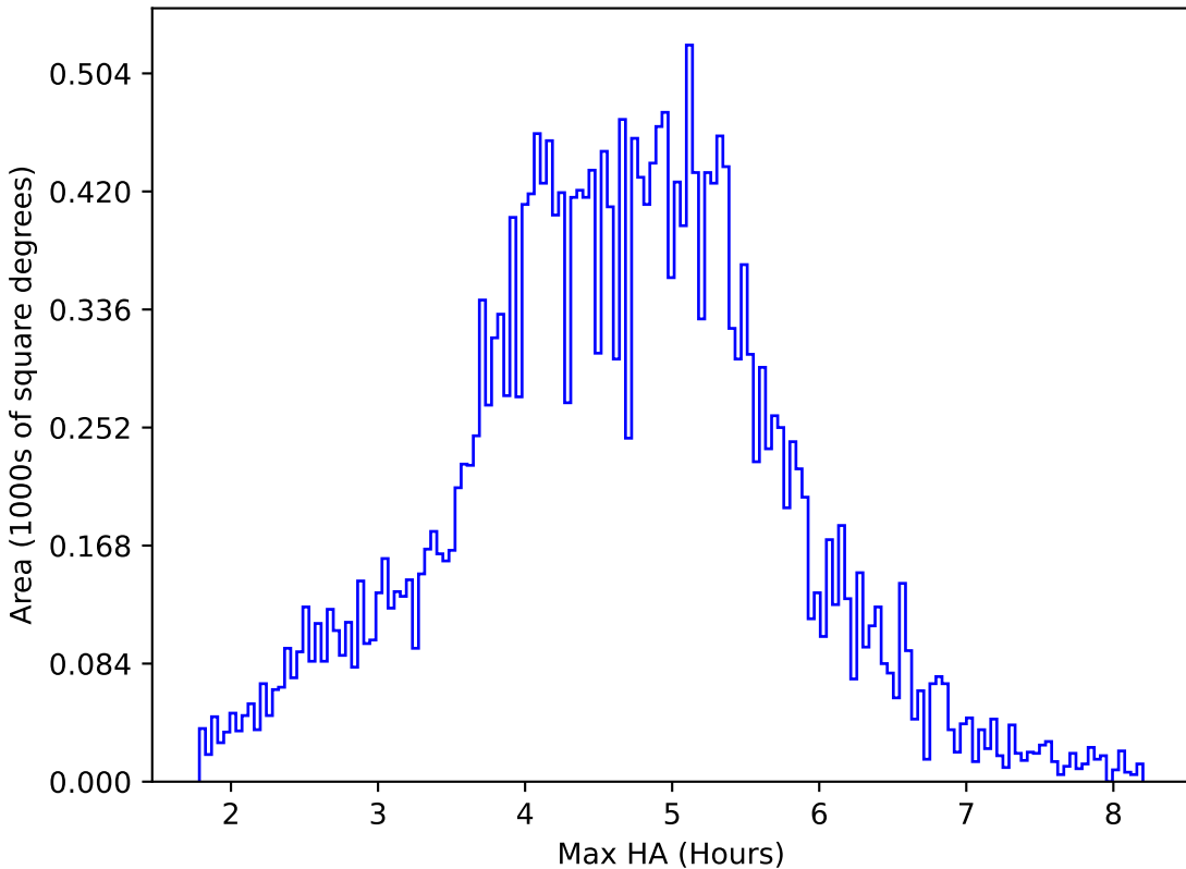
weather_cloudso2v3.4_10yrs All sky i band: Max HA
