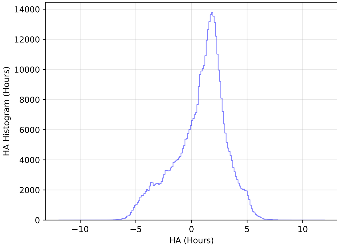
weather_cloudso2v3.4_10yrs WFD z band: HA Histogram
