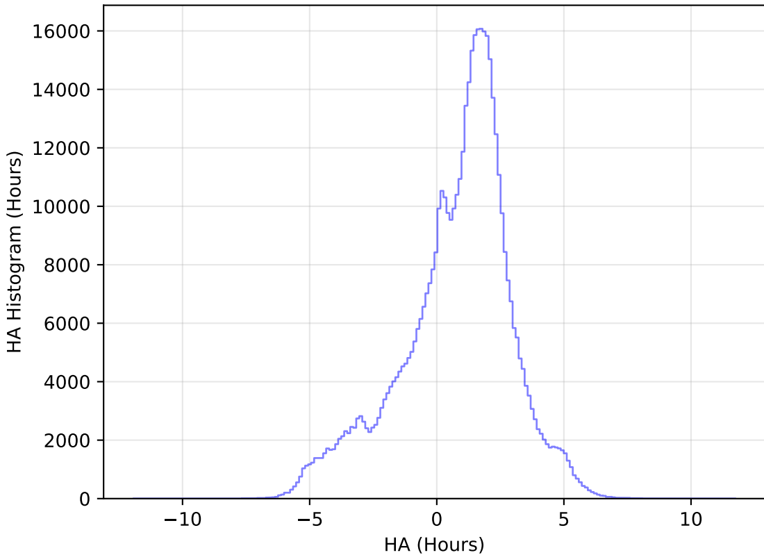
weather_cloudso2v3.4_10yrs WFD i band: HA Histogram
