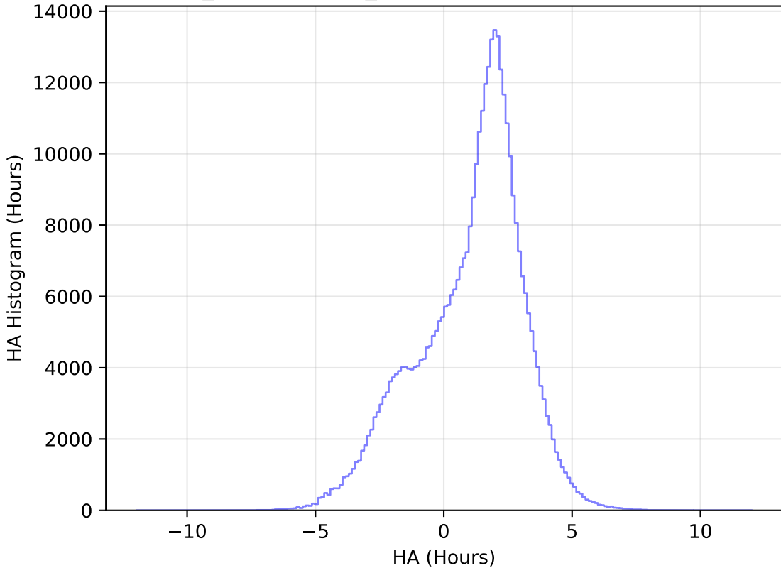
weather_cloudso2v3.4_10yrs All sky y band: HA Histogram
