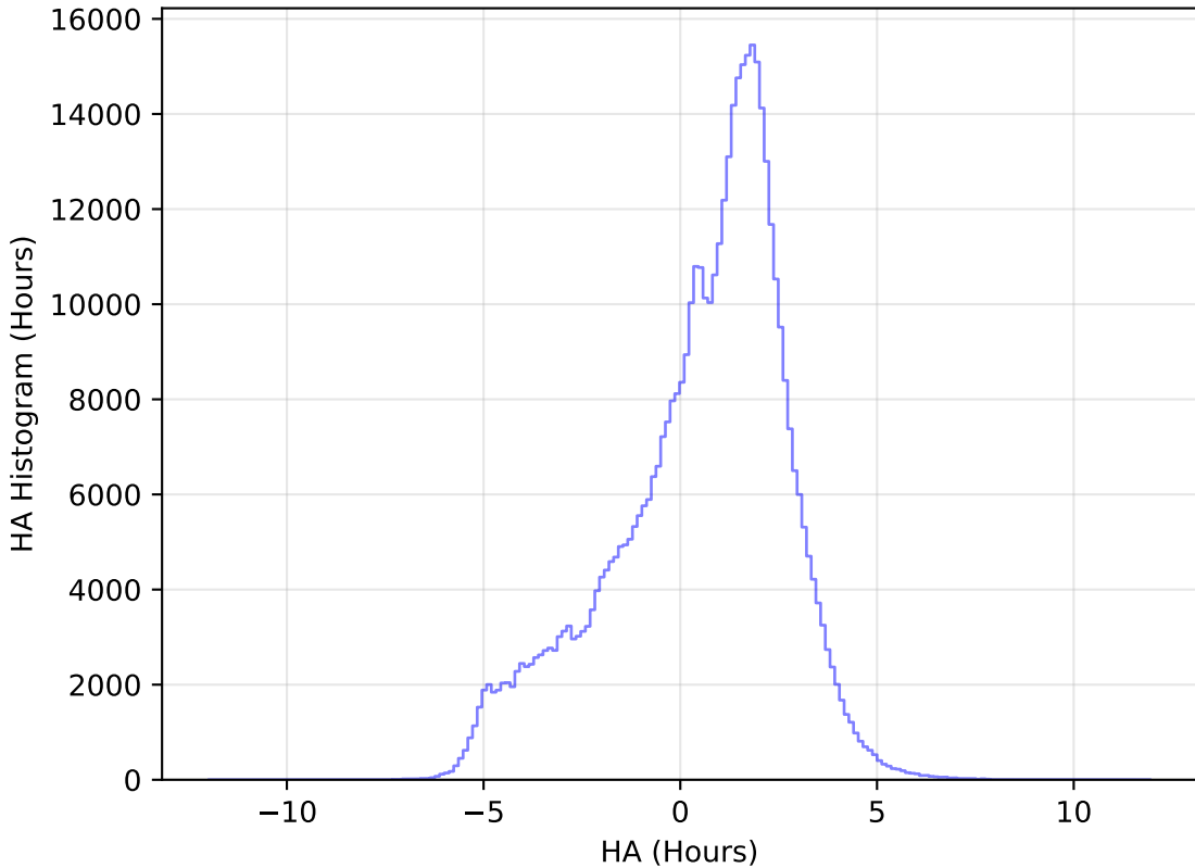
weather_cloudso2v3.4_10yrs All sky r band: HA Histogram
