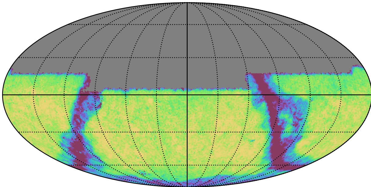
weather_cloudso2v3.4_10yrs Yr 1 y band: Exgal_CoaddM5
