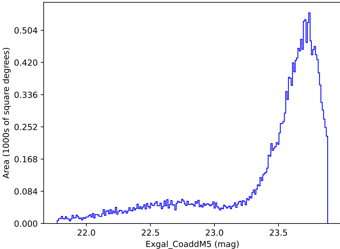
weather_cloudso2v3.4_10yrs Yr 1 y band: Exgal_CoaddM5
