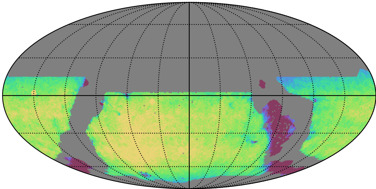
weather_cloudso2v3.4_10yrs WFD y band: Exgal_CoaddM5
