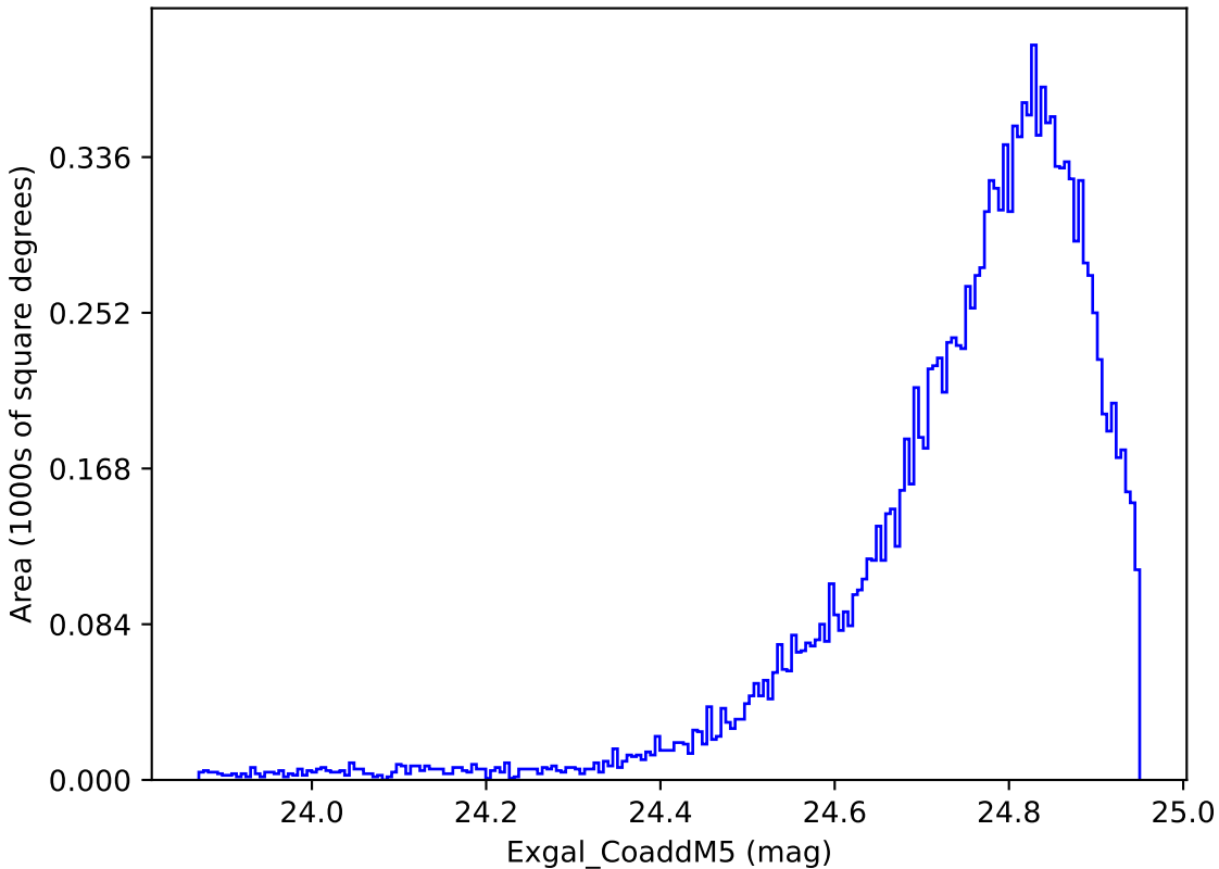
weather_cloudso2v3.4_10yrs WFD y band: Exgal_CoaddM5
