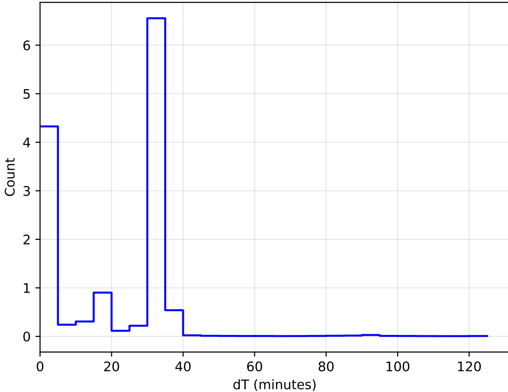
weather_cloudso2v3.4_10yrs All sky: DeltaT Histogram
