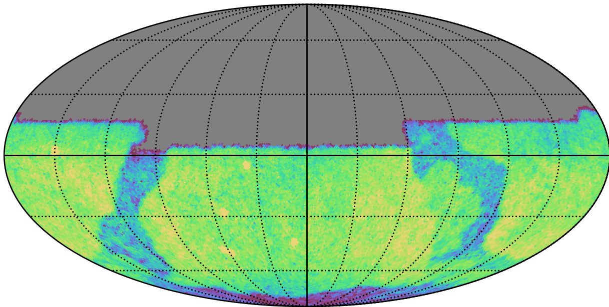
weather_cloudso2v3.4_10yrs Yr 1 y band: CoaddM5
