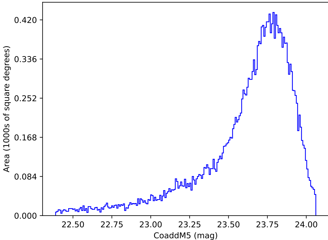
weather_cloudso2v3.4_10yrs Yr 1 y band: CoaddM5
