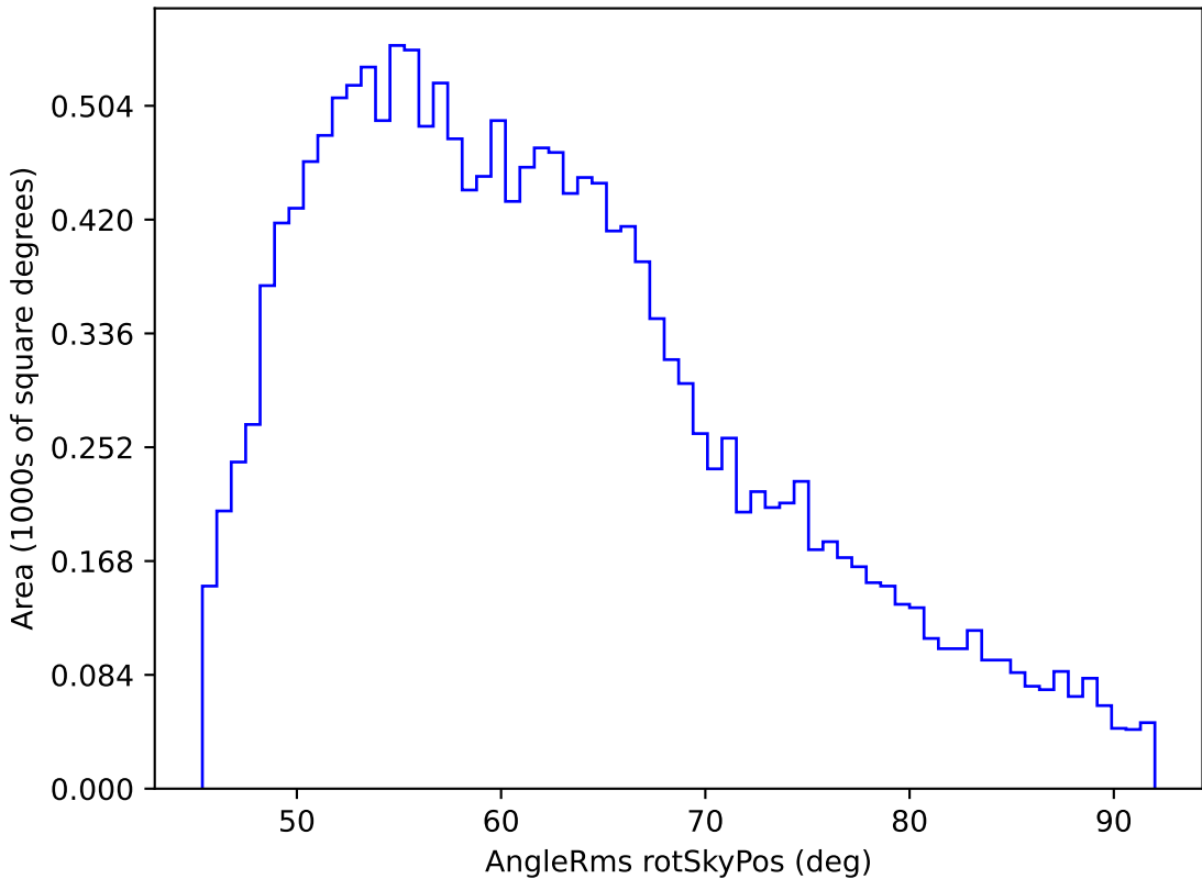
weather_cloudso2v3.4_10yrs WFD y band: AngleRms rotSkyPos
