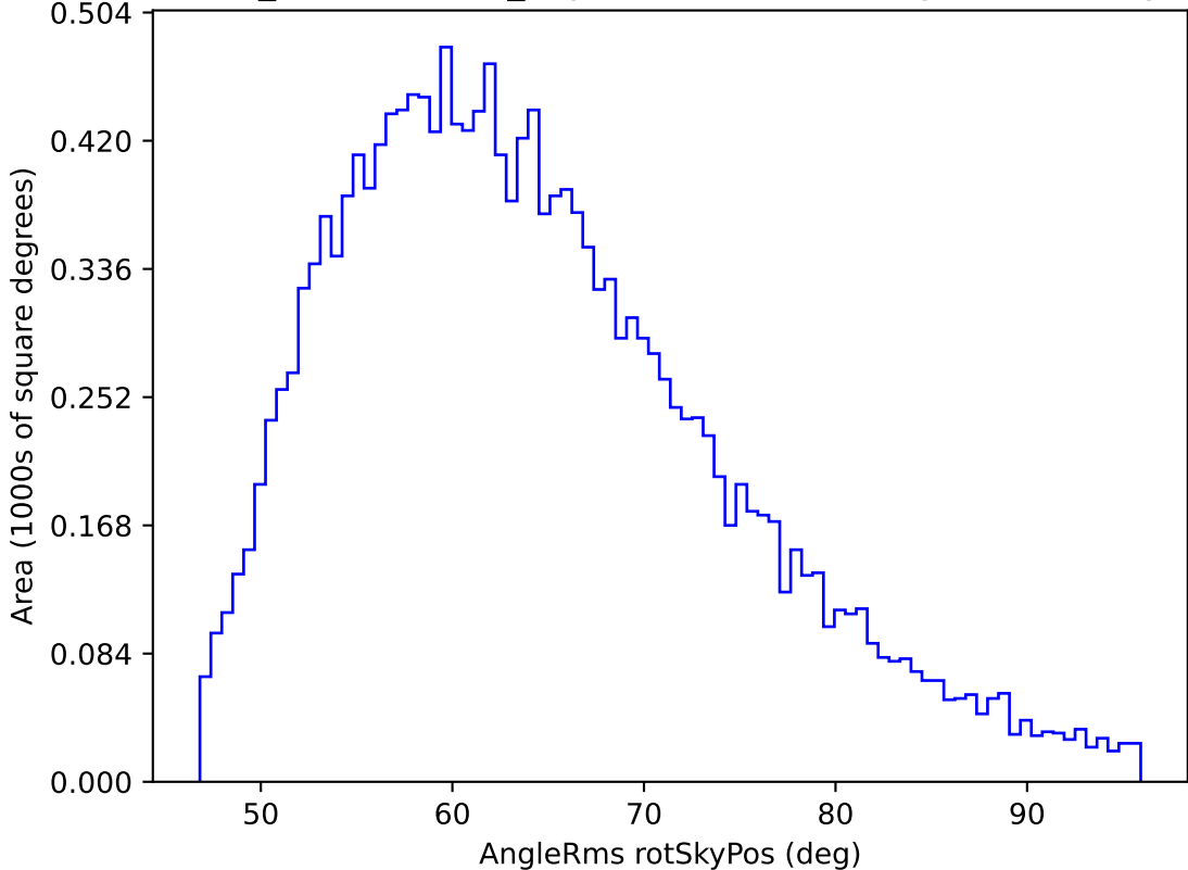
weather_cloudso2v3.4_10yrs WFD u band: AngleRms rotSkyPos
