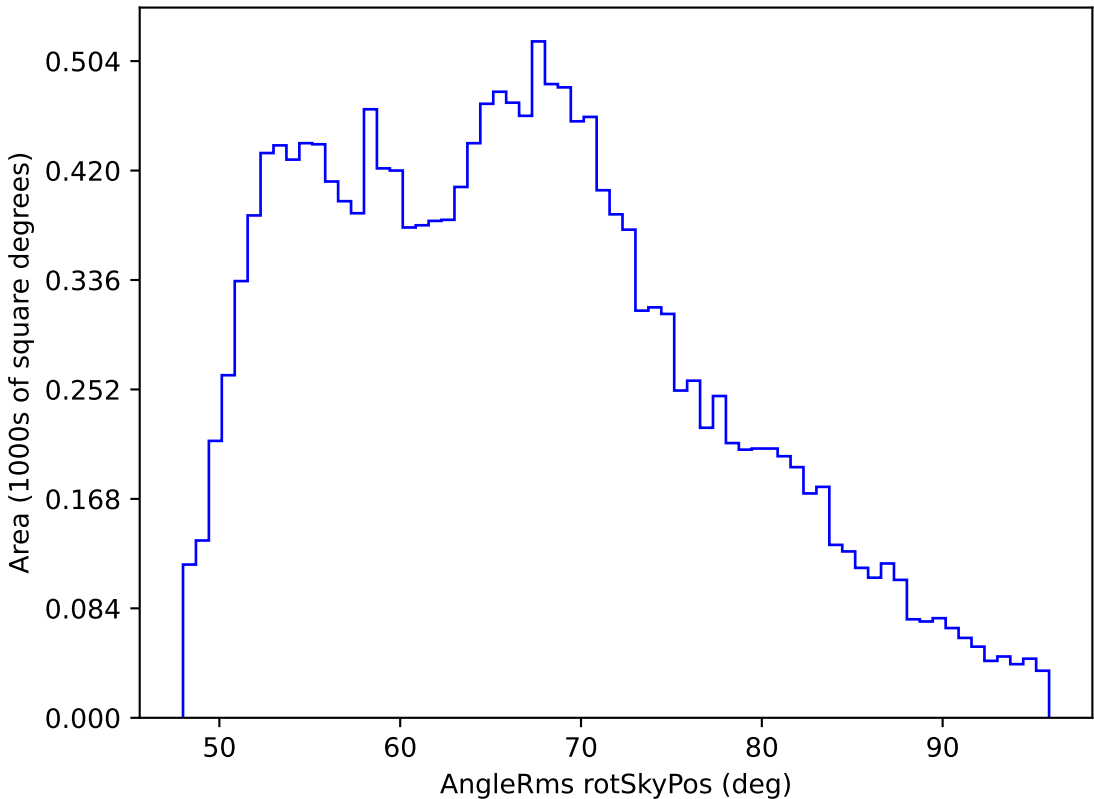
weather_cloudso2v3.4_10yrs WFD r band: AngleRms rotSkyPos
