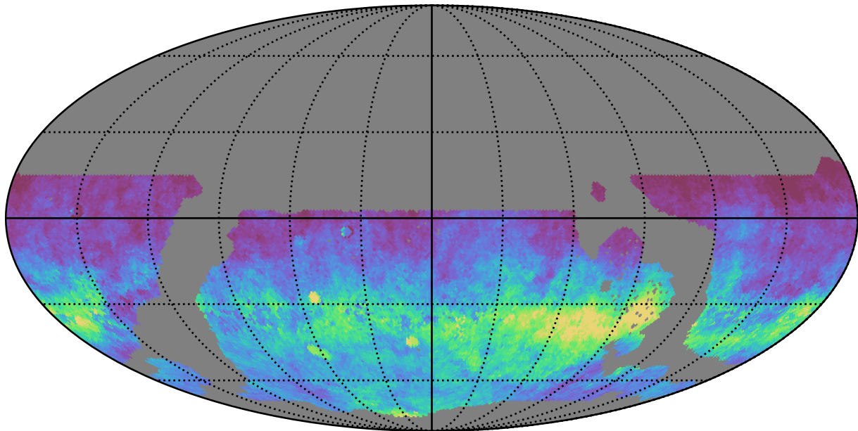
weather_cloudso2v3.4_10yrs WFD i band: AngleRms rotSkyPos
