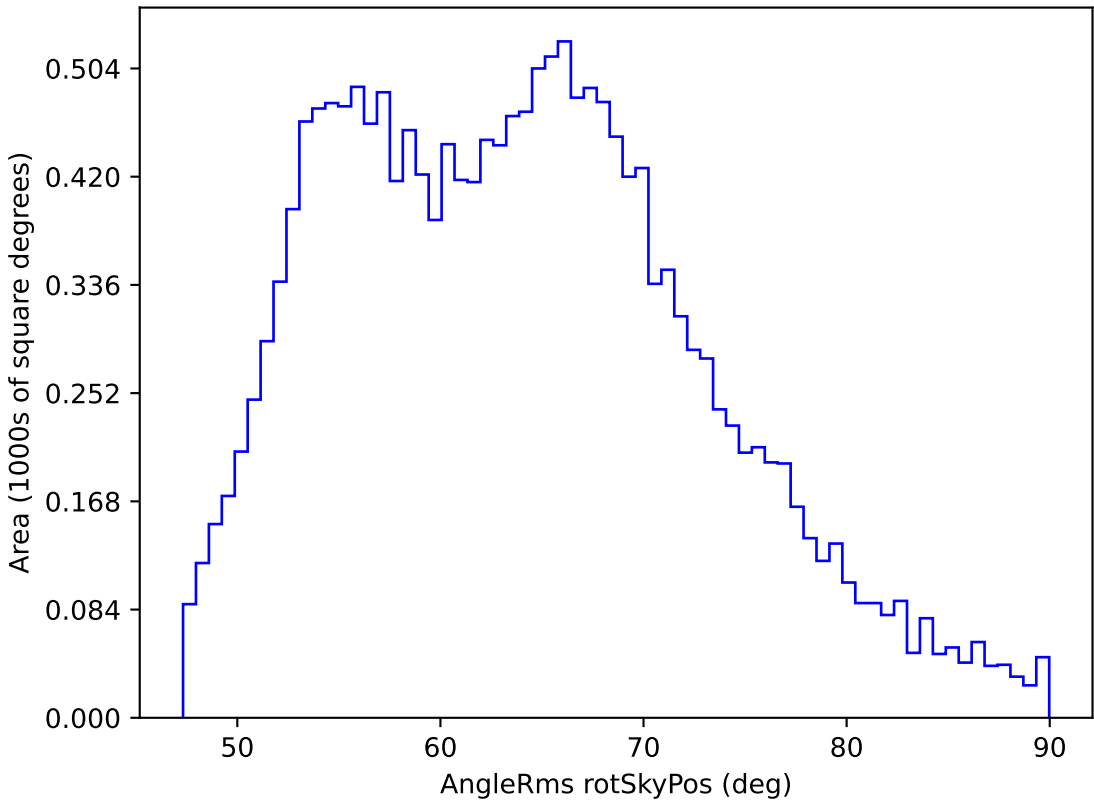
weather_cloudso2v3.4_10yrs WFD i band: AngleRms rotSkyPos
