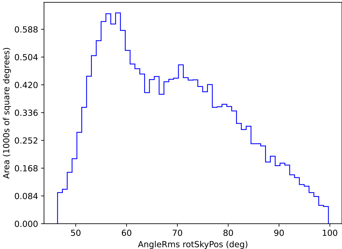
weather_cloudso2v3.4_10yrs WFD g band: AngleRms rotSkyPos
