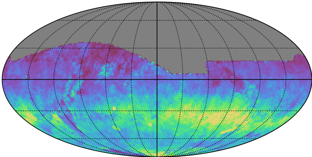
weather_cloudso2v3.4_10yrs All sky z band: AngleRms rotSkyPos
