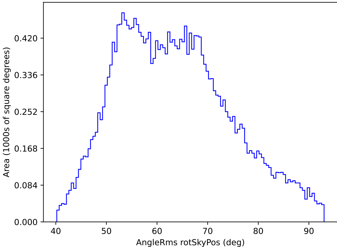
weather_cloudso2v3.4_10yrs All sky z band: AngleRms rotSkyPos
