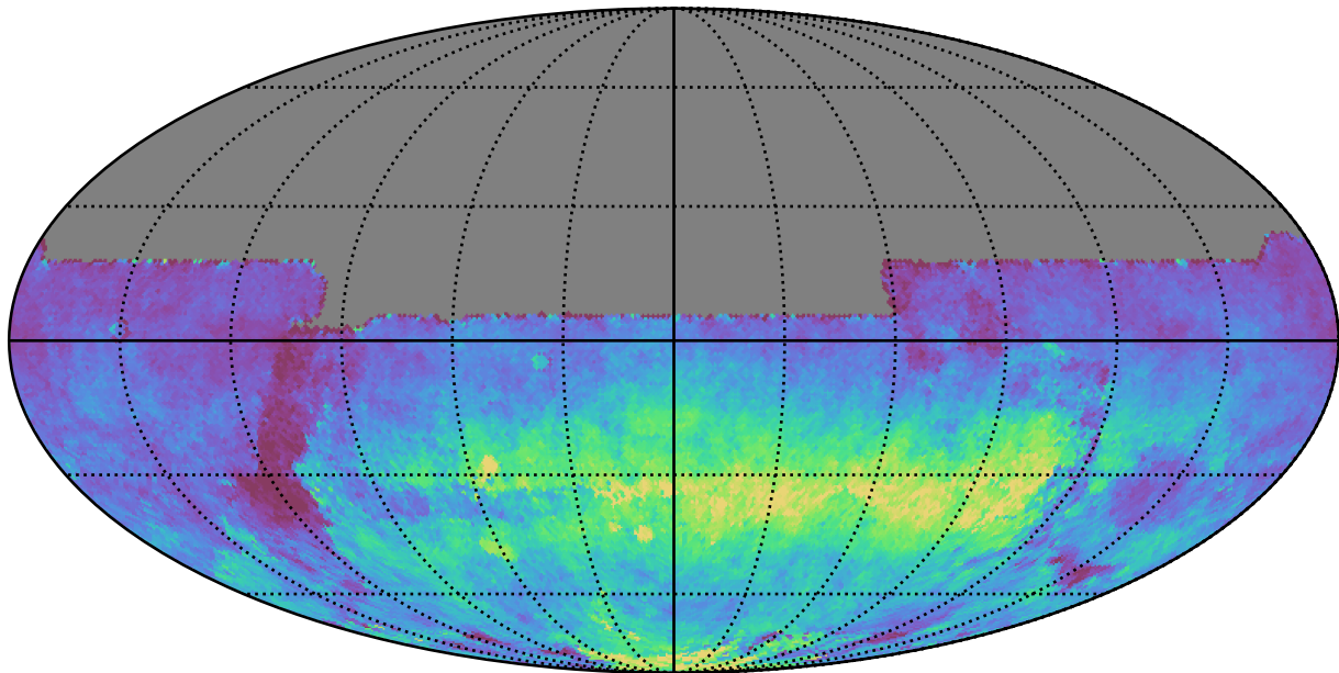
weather_cloudso2v3.4_10yrs All sky y band: AngleRms rotSkyPos
