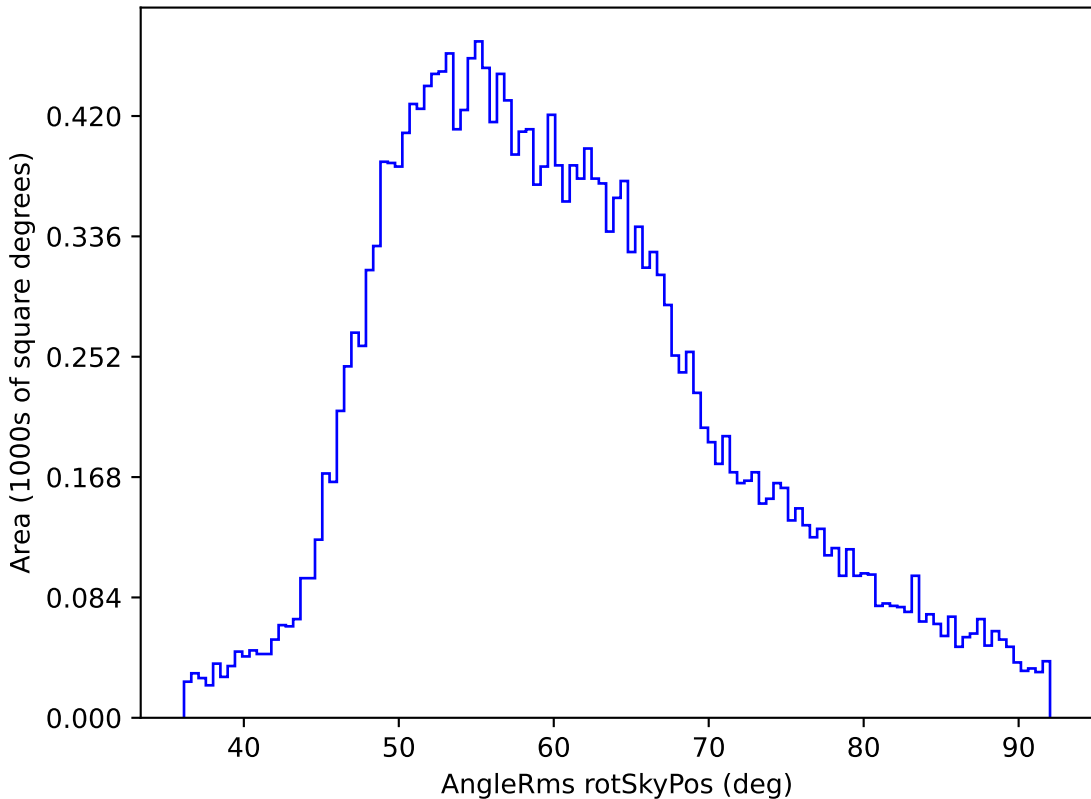
weather_cloudso2v3.4_10yrs All sky y band: AngleRms rotSkyPos
