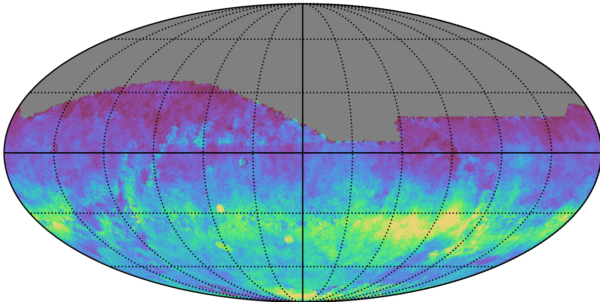
weather_cloudso2v3.4_10yrs All sky i band: AngleRms rotSkyPos
