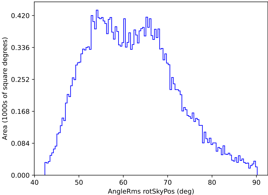
weather_cloudso2v3.4_10yrs All sky i band: AngleRms rotSkyPos
