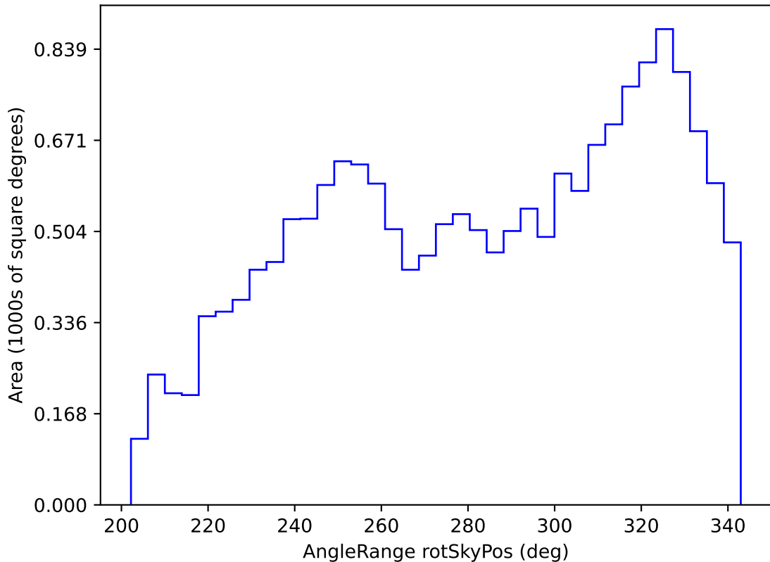
weather_cloudso2v3.4_10yrs WFD z band: AngleRange rotSkyPos
