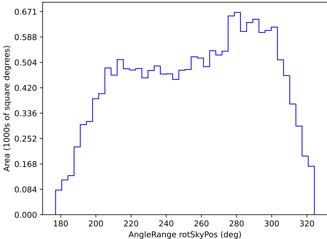
weather_cloudso2v3.4_10yrs WFD u band: AngleRange rotSkyPos
