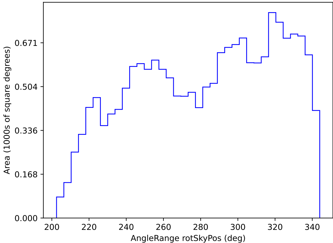
weather_cloudso2v3.4_10yrs WFD r band: AngleRange rotSkyPos
