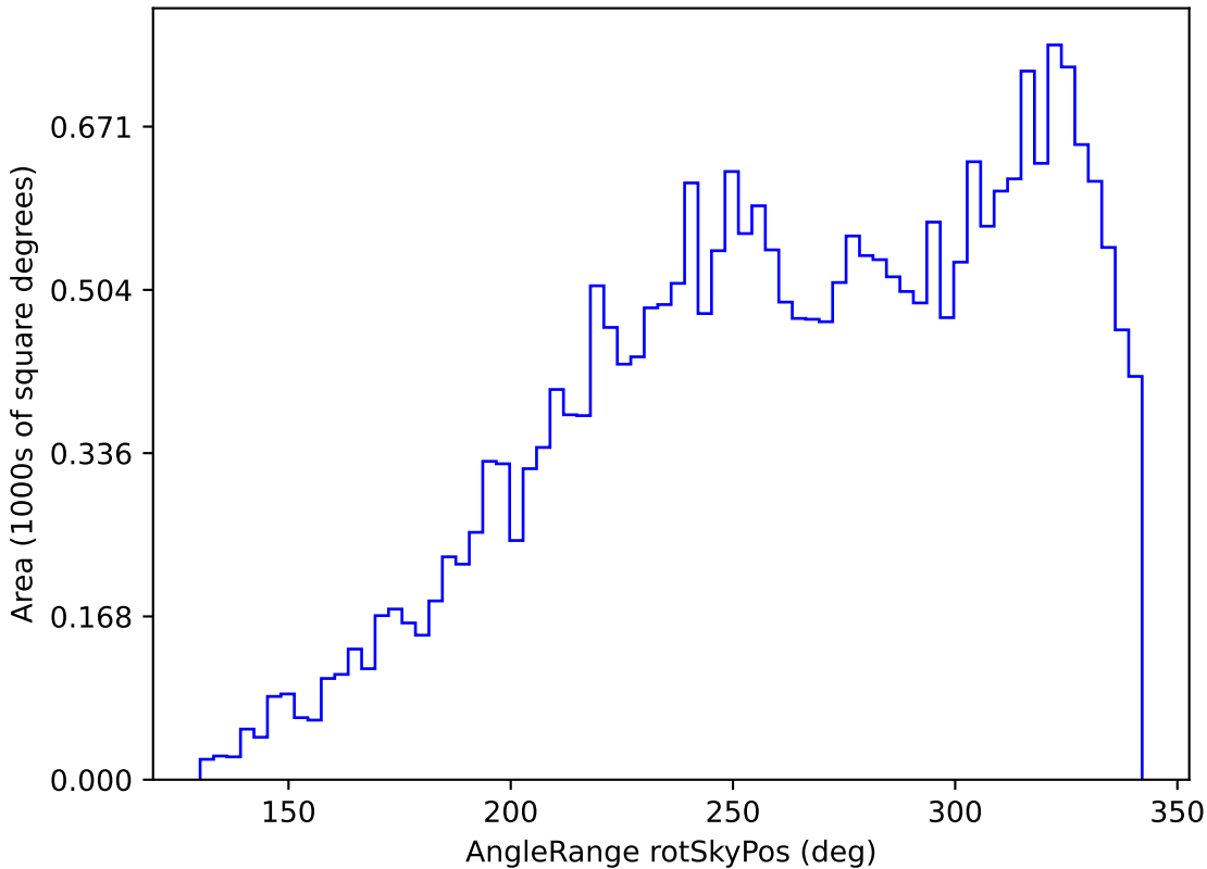
weather_cloudso2v3.4_10yrs All sky z band: AngleRange rotSkyPos
