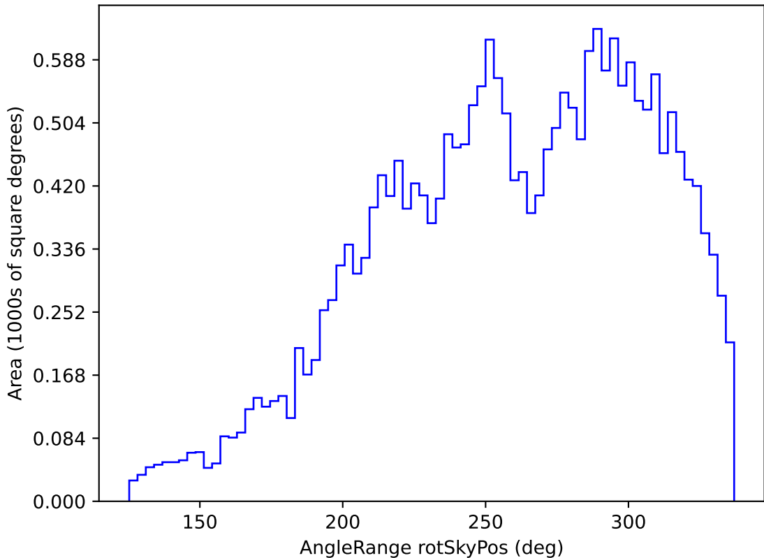
weather_cloudso2v3.4_10yrs All sky y band: AngleRange rotSkyPos
