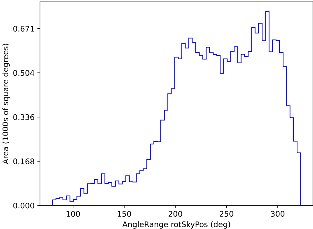
weather_cloudso2v3.4_10yrs All sky u band: AngleRange rotSkyPos
