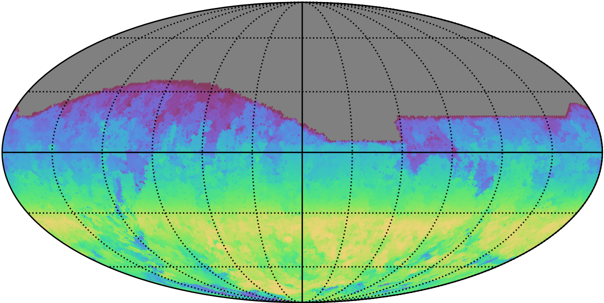
weather_cloudso2v3.4_10yrs All sky i band: AngleRange rotSkyPos
