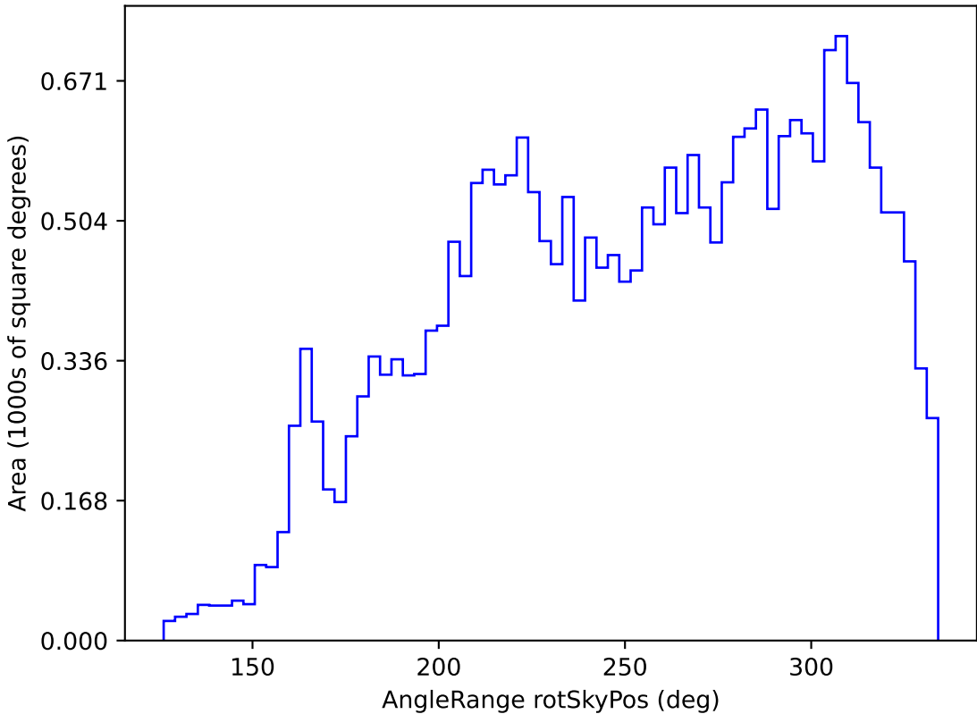
weather_cloudso2v3.4_10yrs All sky g band: AngleRange rotSkyPos
