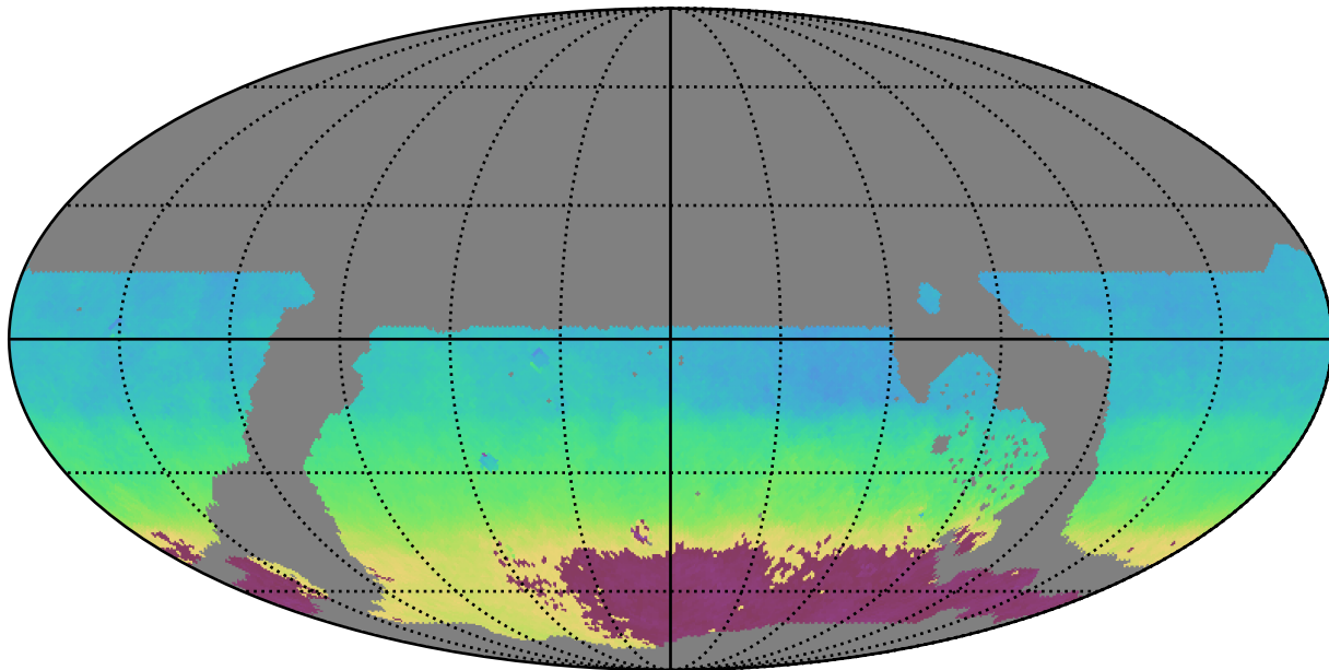
weather_cloudso2v3.4_10yrs WFD z band: AngleMean rotSkyPos
