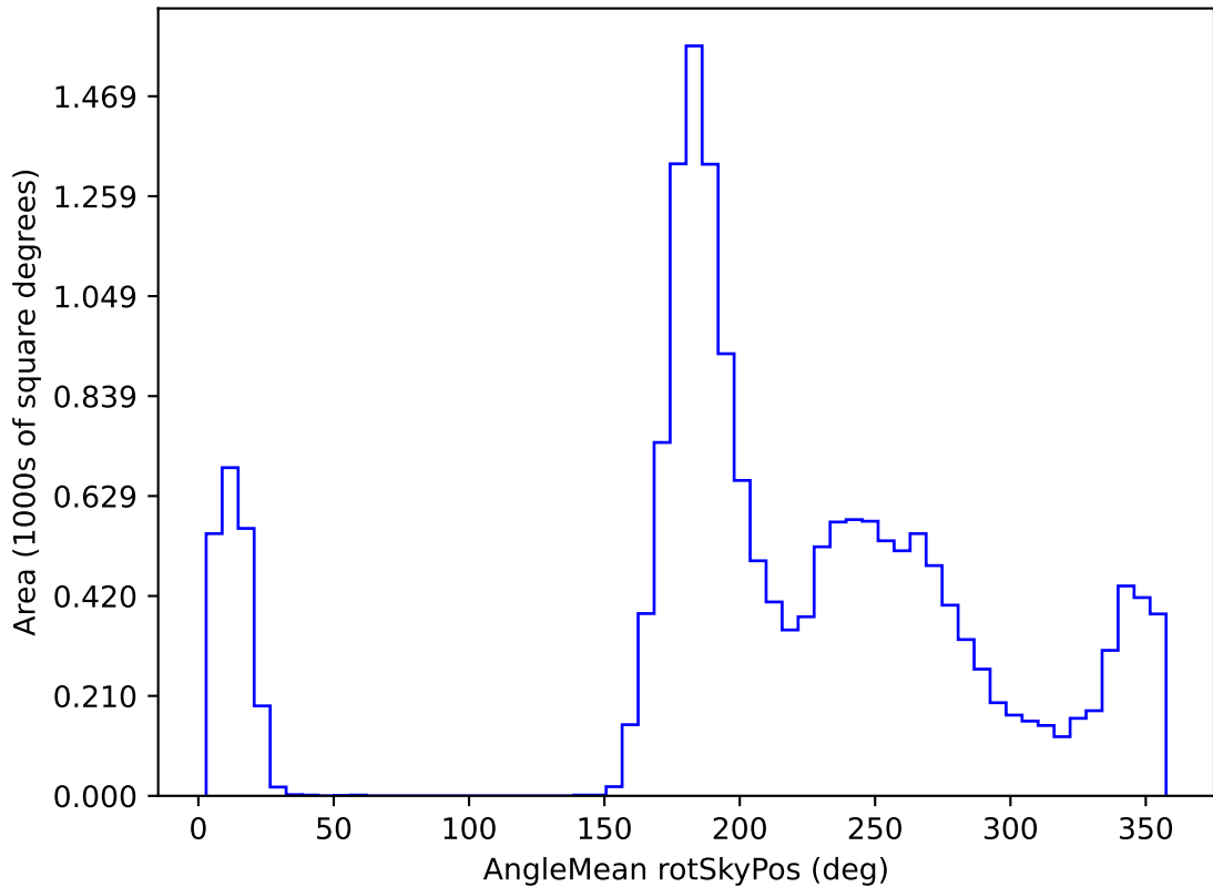
weather_cloudso2v3.4_10yrs WFD z band: AngleMean rotSkyPos
