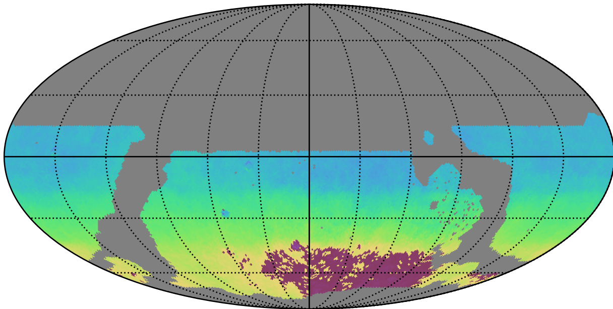
weather_cloudso2v3.4_10yrs WFD y band: AngleMean rotSkyPos
