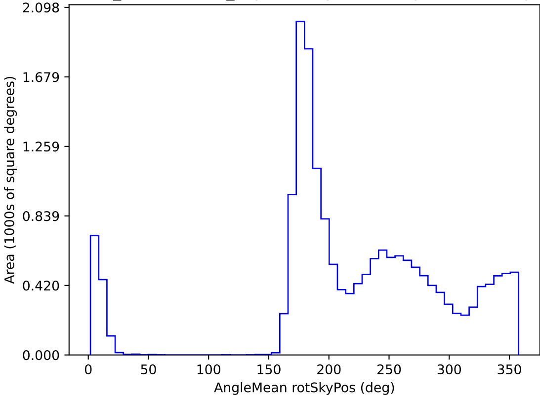
weather_cloudso2v3.4_10yrs WFD y band: AngleMean rotSkyPos
