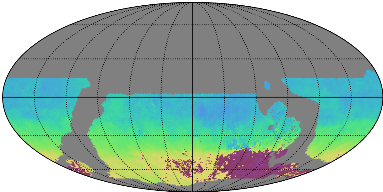
weather_cloudso2v3.4_10yrs WFD u band: AngleMean rotSkyPos
