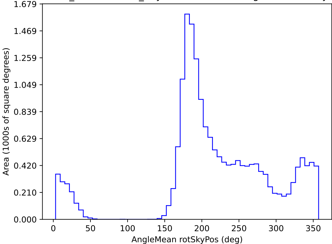
weather_cloudso2v3.4_10yrs WFD u band: AngleMean rotSkyPos
