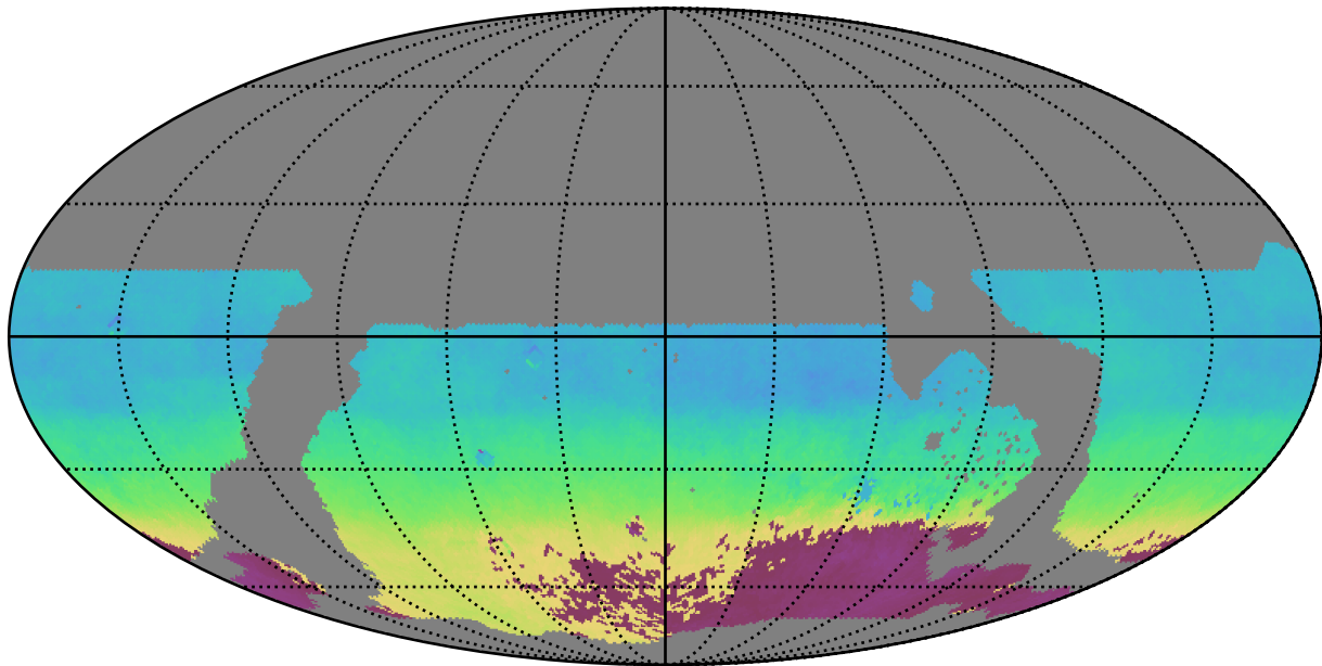
weather_cloudso2v3.4_10yrs WFD r band: AngleMean rotSkyPos
