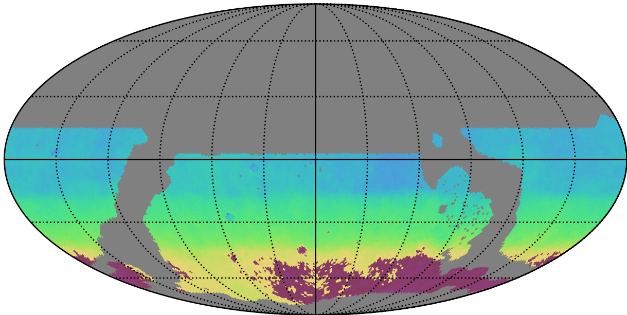
weather_cloudso2v3.4_10yrs WFD i band: AngleMean rotSkyPos
