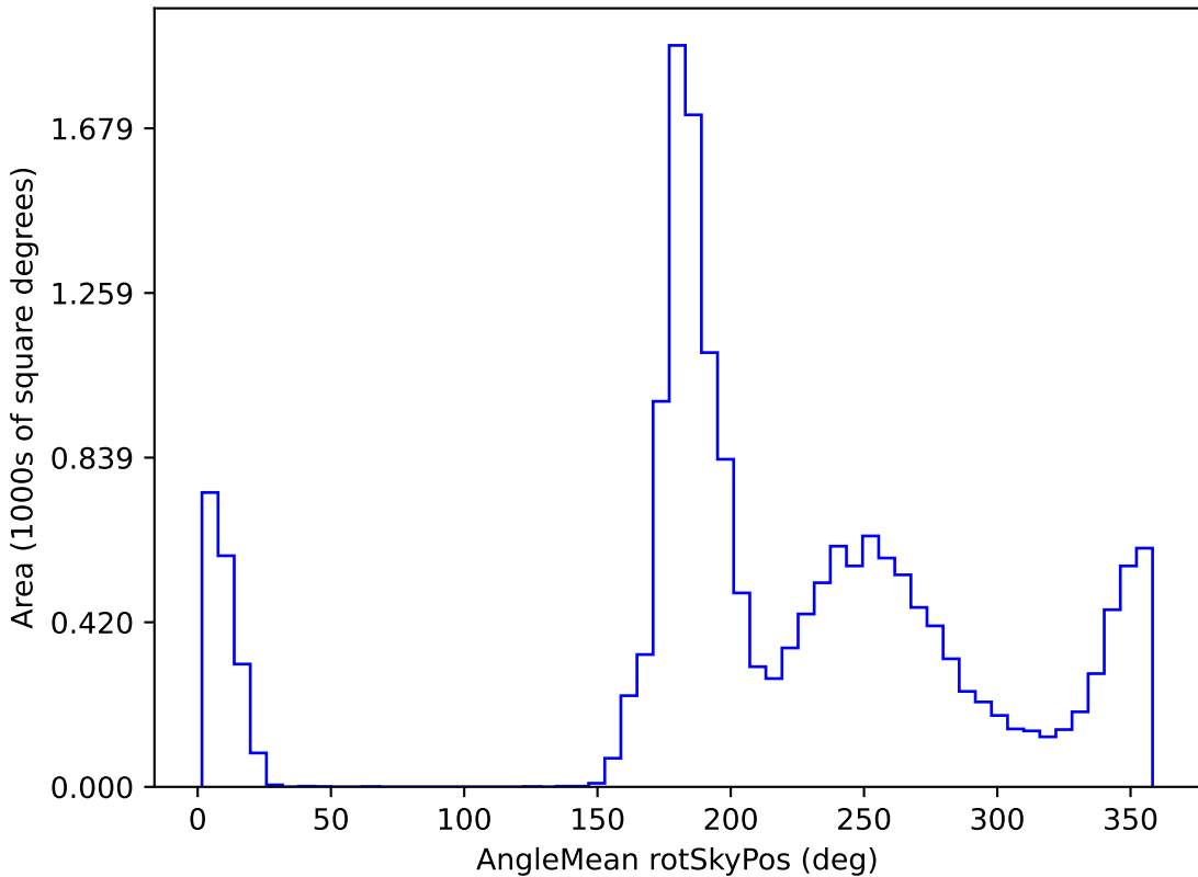
weather_cloudso2v3.4_10yrs WFD i band: AngleMean rotSkyPos
