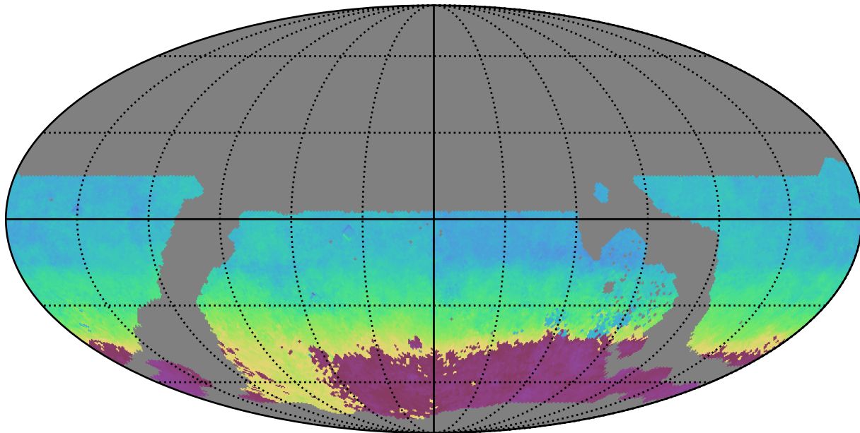
weather_cloudso2v3.4_10yrs WFD g band: AngleMean rotSkyPos
